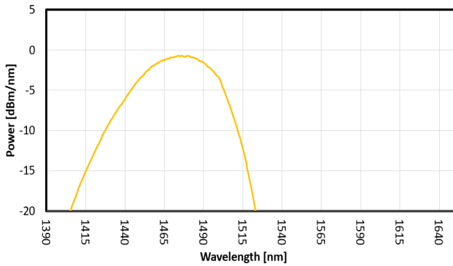
FIG. 3: SLED 2 SPECTRUM
