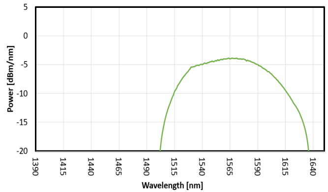
FIG. 2: SLED 1 SPECTRUM
