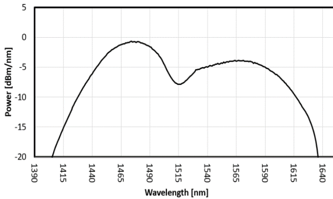
FIG. 1: OSE2 SPECTRUM
