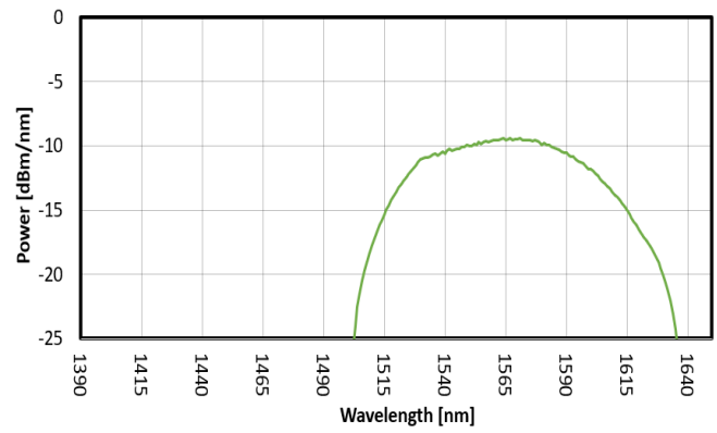
FIG. 2: SLED 1 SPECTRUM
